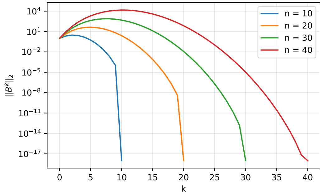
\|B^k\|_2 (transitorio)
